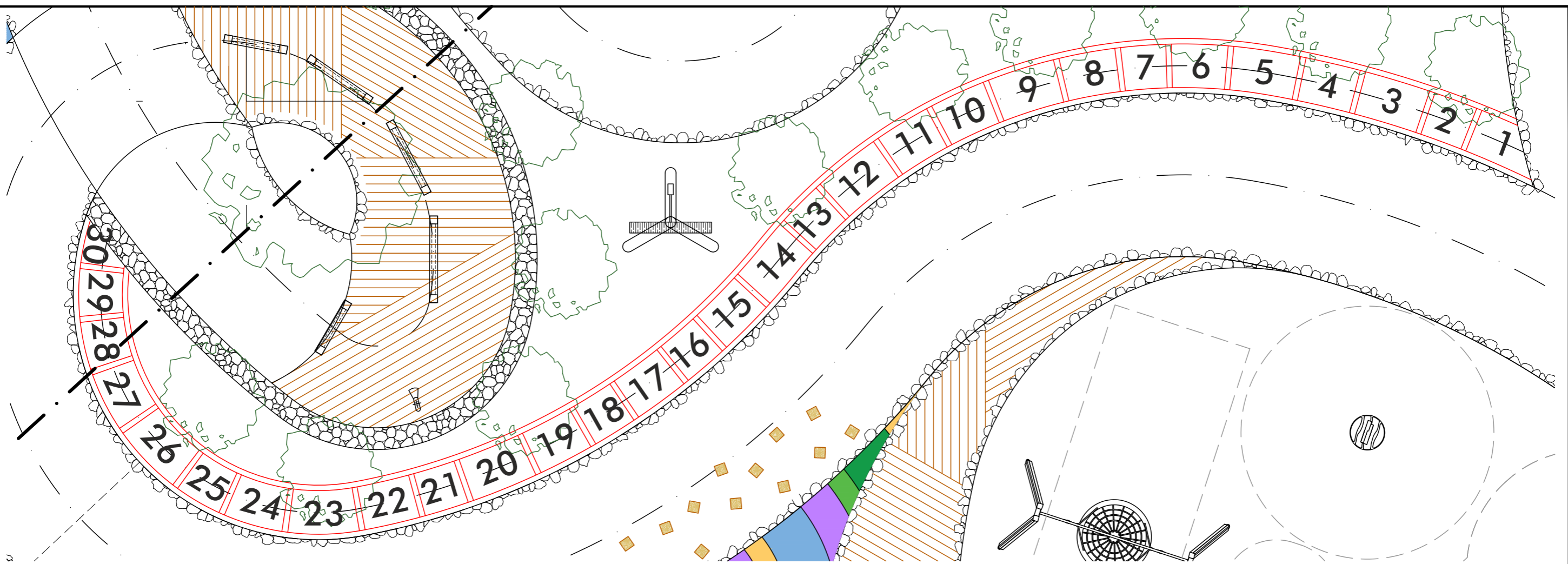
PLANTA DE RECORRIDO SENSORIAL Escala 1/75
