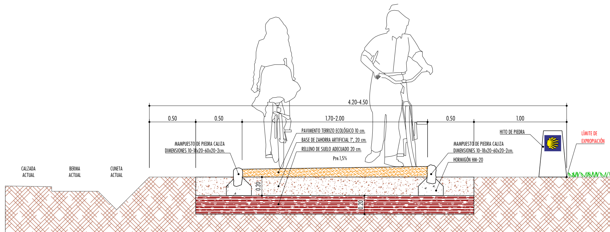
SECCIÓN TIPO ejes 1, 2 y 3 (carril bici en zona rústica) Escala 1/25
